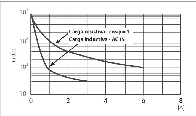
F 7S14 - Vida útil eléctrica (AC) en función de la carga - 7S.14/34
