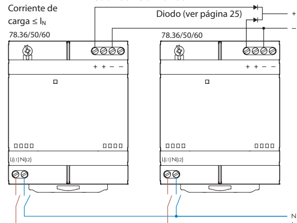
Redundancia manual
