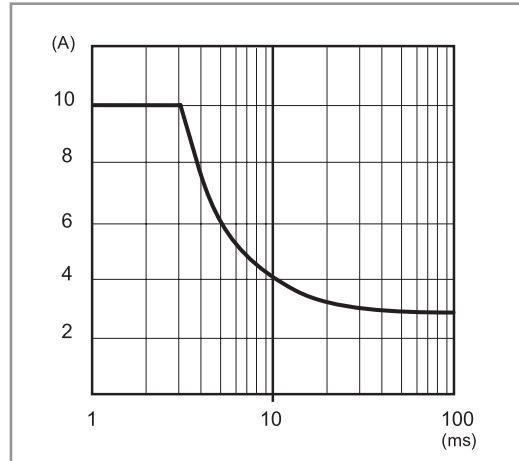
P78-5 Pico de corriente de salida en función del tiempo (78.50)
