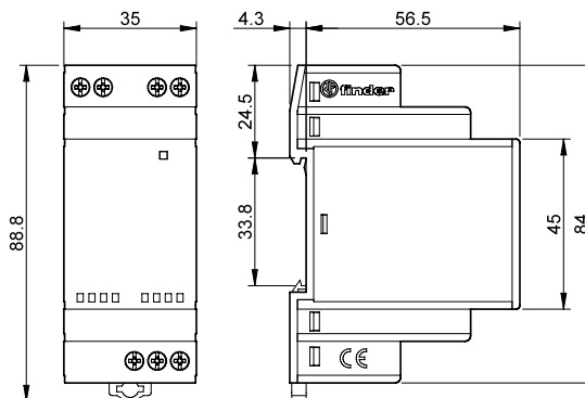
Tipo 78.50 / 78.60 Borne de jaula
