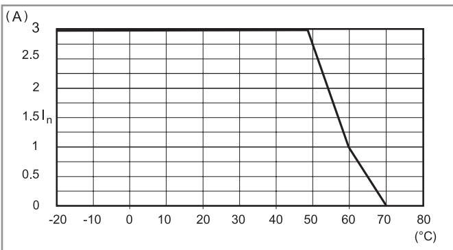
L78-3 Corriente de salida en función de la temperatura ambiente (78.36) - 12 V
