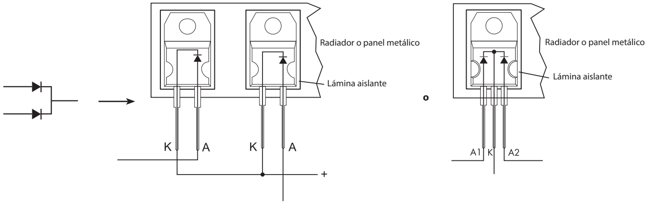
Diode para los tipos 78.25, 78.36, 78.50, 78.60
