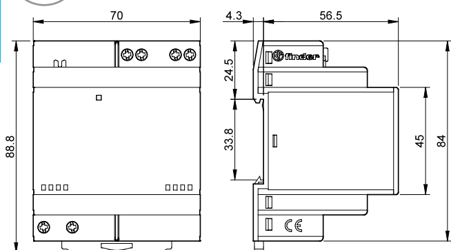
Tipo 78.1B Borne de jaula
