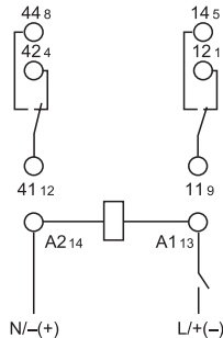
Esquema de conexión (sin señal de mando)
