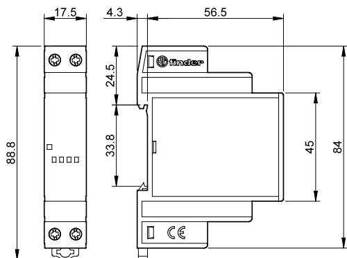
Tipo 78.36 Borne de jaula
