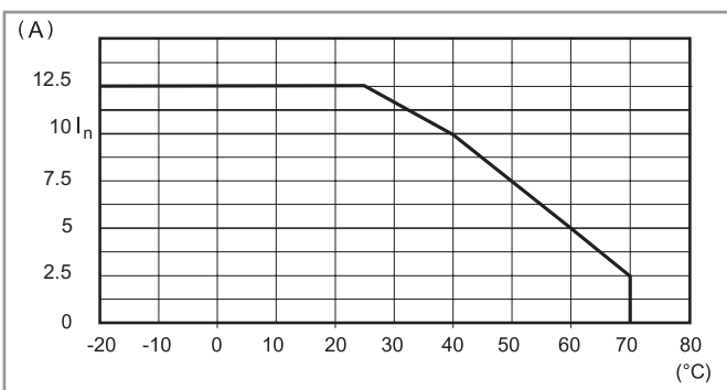
L78-11 Corriente de salida en función de la temperatura ambiente (78.2E)
