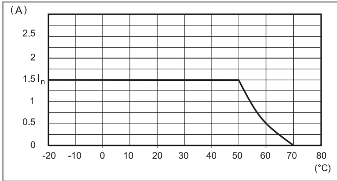
L78-3 Corriente de salida en función de la temperatura ambiente (78.36) - 24 V
