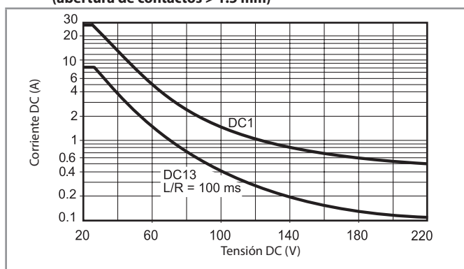
H 66 - Máxima capacidad de corte en DC, ejecuciones x60x (abertura de contactos > 1.5 mm)
