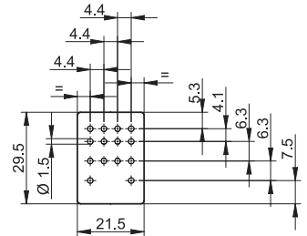
Vista parte inferior
