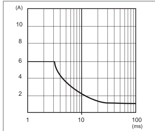
P78-4 Pico de corriente de salida en función del tiempo (78.60)
