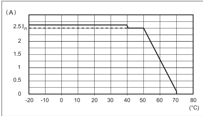
L78-4 Corriente de salida en función de la temperatura ambiente (78.60)
