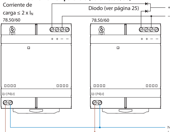
Conexión en paralelo (solo 78.50/60)
