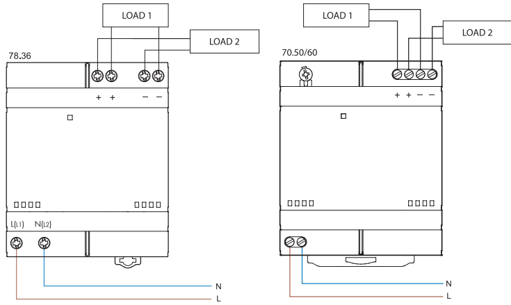
Conexión dual
