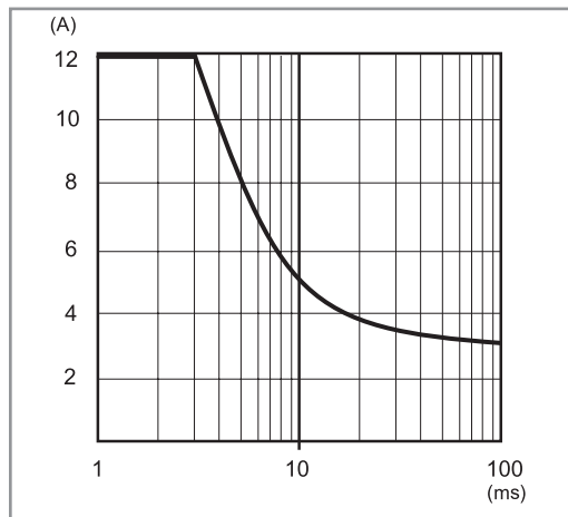
P78-3 Pico de corriente de salida en función del tiempo (78.36) - 12 V
