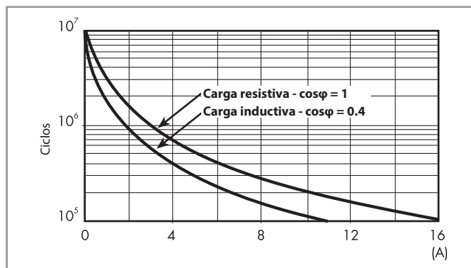
F 46 - Vida eléctrica (AC) en función de la corriente de contactos
