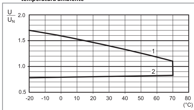
R 66 - Campo de funcionamiento de la bobina AC en función de la temperatura ambiente
