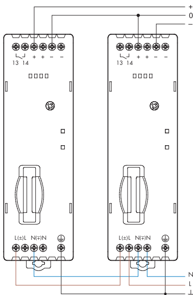
Conexión dual
