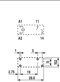
Vista parte inferior
