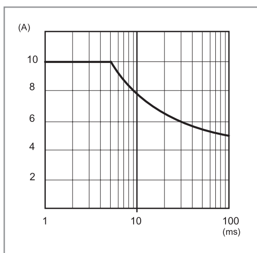
P78-8 Pico de corriente de salida en función del tiempo (78.1B)
