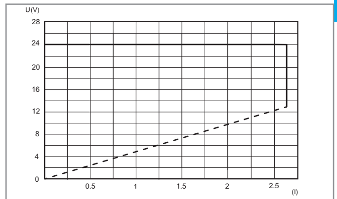
FB78-2 Tensión de salida en función de la corriente de salida (78.60)
